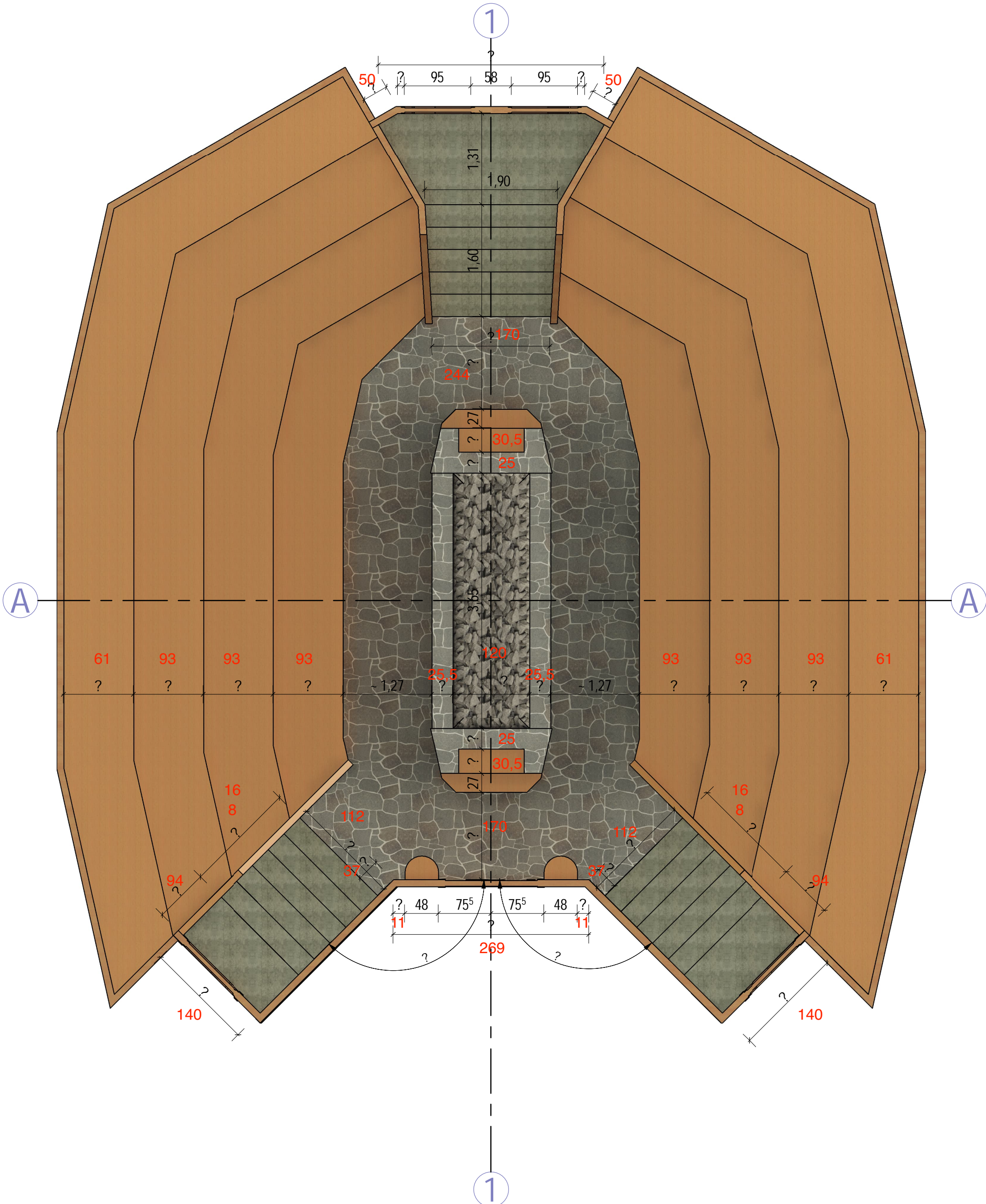
Grundriss Satama 1 : 50
